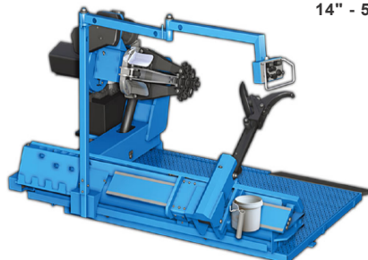
MÁQUINA DESMONTAR/MONTAR PNEUS ECF 356 PESADOS
