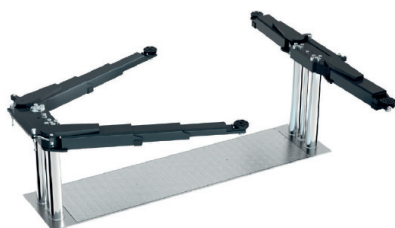
ELEVADOR HIDRÁULICO DUPLO PISTÃO - 5.5T. REF: 2055/L .....
